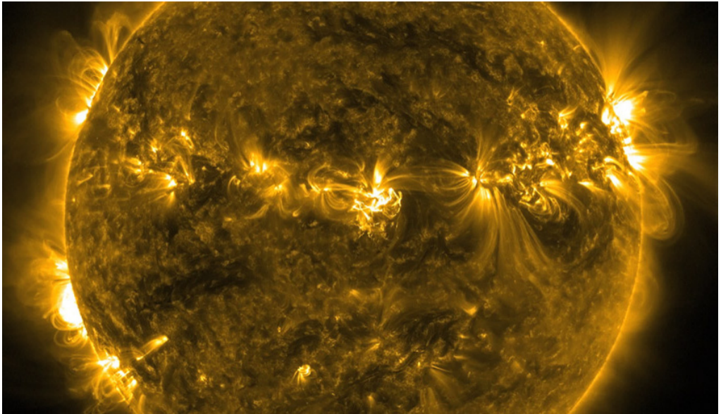
SDO/NASA, EUV: 28/09/2011 – 02/10/2011
